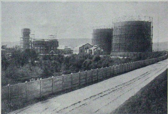
A nagy gáztartók, az épülő víztorony és kátránymedencék.
