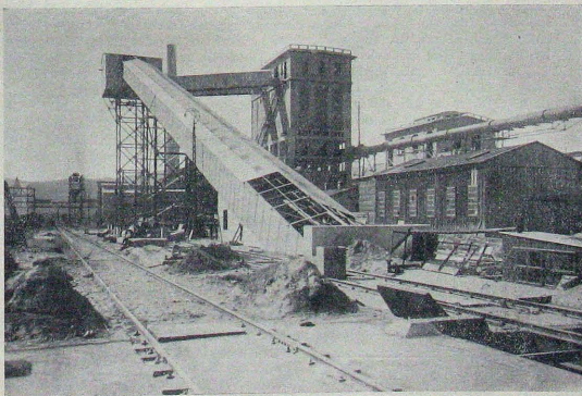
A fővárosi gázugyár építkezése. — A széntorony és szén szállító berendezés.
