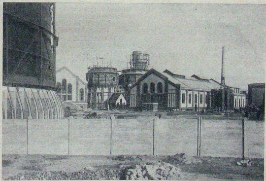
A fővárosi új gázugyár építkezése. — A gáztisztító épület és kátránytartók.
