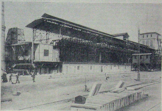
A fővárosi új gázipart építkezése. — A gázfejlesztő kemencék.
