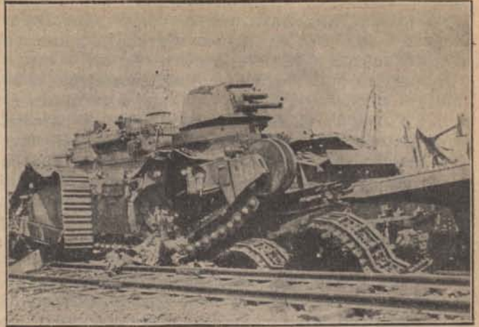
Ezt a 72 tonnás legnehezebb fajtájú (francia) harcokocsit a németek még a szállító vasúti aljazaton lőtték szét.
